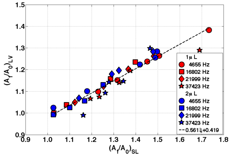
Figura 8. Cociente entre el área final e inicial de la interface líquido-vapor como función del cociente entre el área final e inicial de la interface sólido-líquido de una gota de agua de 1.0 y 2.0 [μl] para 4 diferentes frecuencias.
