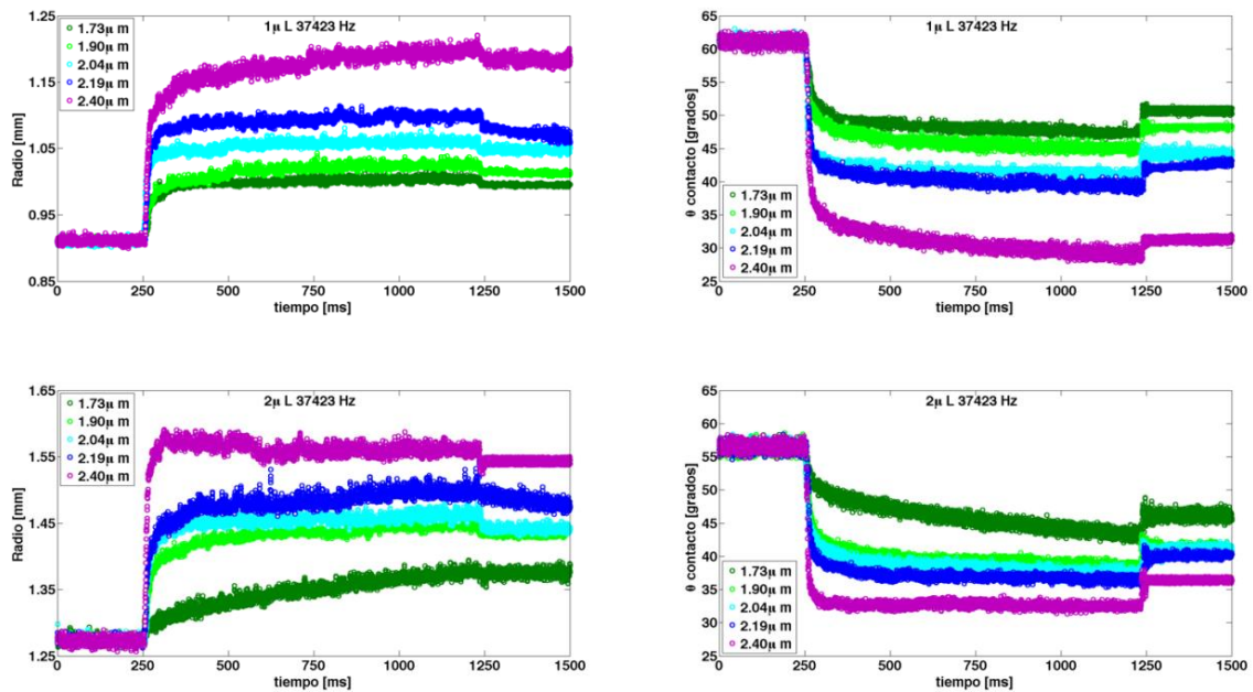
Figura 6. Evolución temporal del radio y ángulo de contacto de una gota de agua de 1.0 y 2.0 [μl] depositada sobre un sustrato sólido al aplicar vibraciones verticales a 37423 [Hz].
