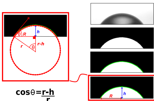
Figura 2. Esquema del método de detección del ángulo de contacto, radio de
