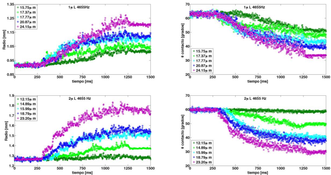
Figura 5. Evolución temporal del radio y ángulo de contacto de una gota de agua de 1.0 y 2.0 [ \mu\text{l} ] depositada sobre un sustrato sólido al aplicar vibraciones verticales a 4655 [Hz].
