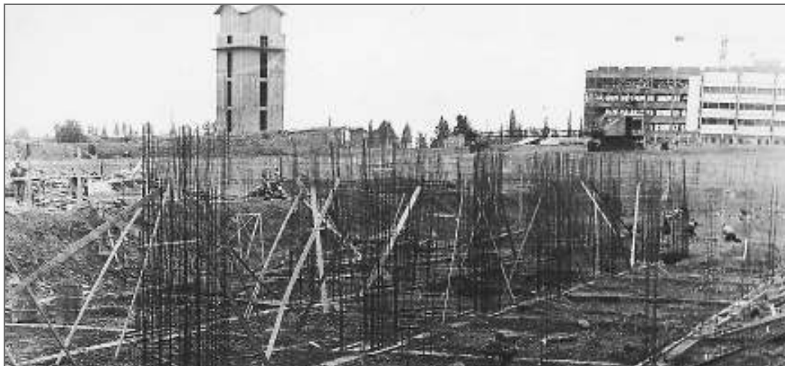
Inicio de la construcción del edificio de Ciencias Políticas y Sociales (cimientos y arranque de columnas). Según consta en el Informe, figura en obras en ejecución en 1969. En la parte superior, la estructura de la torre de agua del ex Hospital de Niños. A la derecha, la continuidad de la construcción de la Facultad de Ciencias Económicas.
